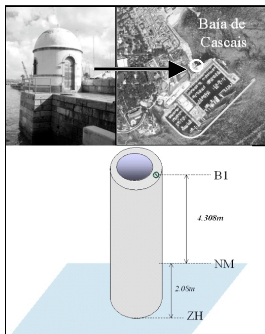
Fig. 1 - Marégrafo de Cascais e medição do nível médio do mar. Localização do marégrafo e esboço do poço e respectivas marcas de referência. B1-Marca de nivelamento que serve de referência ao NM (nível médio adoptado; designado nível médio cartográfico ou zero cartográfico); ZH-Zero hidrográfico.
